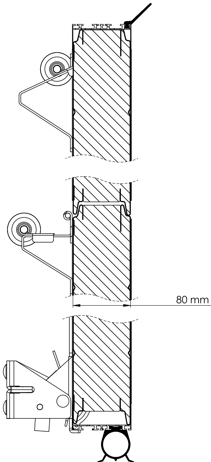
COUPE A-A ECHELLE 1 : 3
