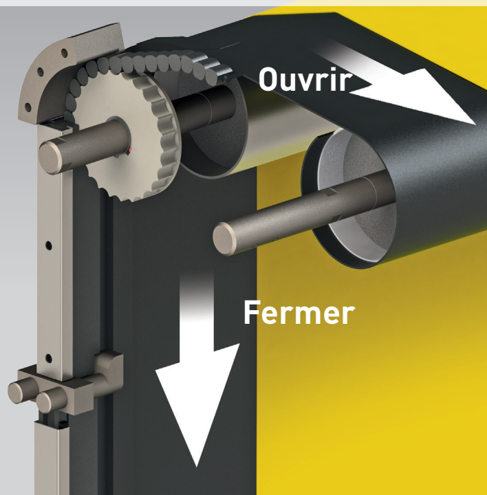
Technologie d'entraînement "PUSH-PULL PT "
